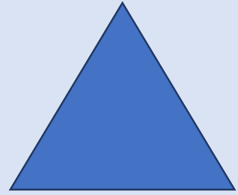
Triangle équilatéral
