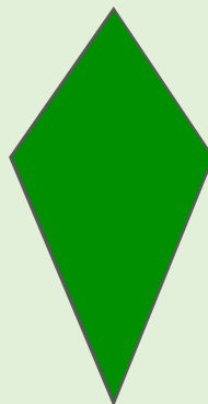
Cerf-volant
