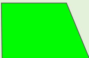
Trapèze rectangle
