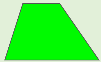
Trapèze quelconque
