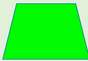
Trapèze isocèle
