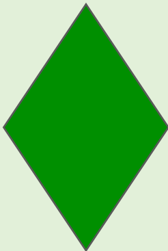
Losange
