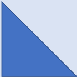
Triangle isocèle rectangle
